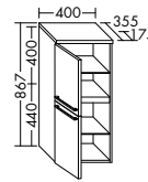
UHBG040/UHBH040
